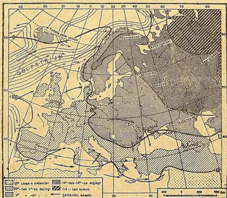
Европаның қышқар ајындағы температурасы мен çели 0° изотерманың Терістік Музды океаннан Қара теңізге қарай ојысьр тусьвннің себеві не?
