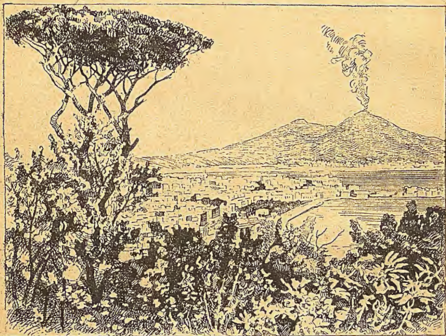
Bezuviј tavь men Neapol. Vulканның тьпыс тuroqandaқысь. Төвенің sol қаюьнда—Somma (eski kraterdiң ceti) tur. Bergi қаюьнда тuroqan аюас- rijnija (Ijtalija қарақажь).
