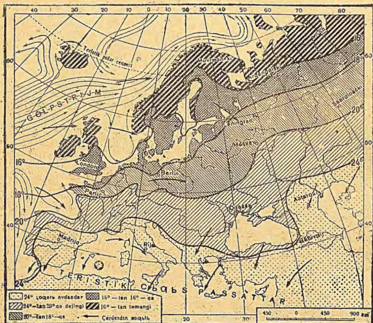
Европаның ужел айнадағы авасы мен Ҷелдериниң температурасы. 20° изотерма Батыс Европадағы 40—параллелден Сыбыс Европаның 50—параллеліне көтеріледі, туньд сеवेбі не?
