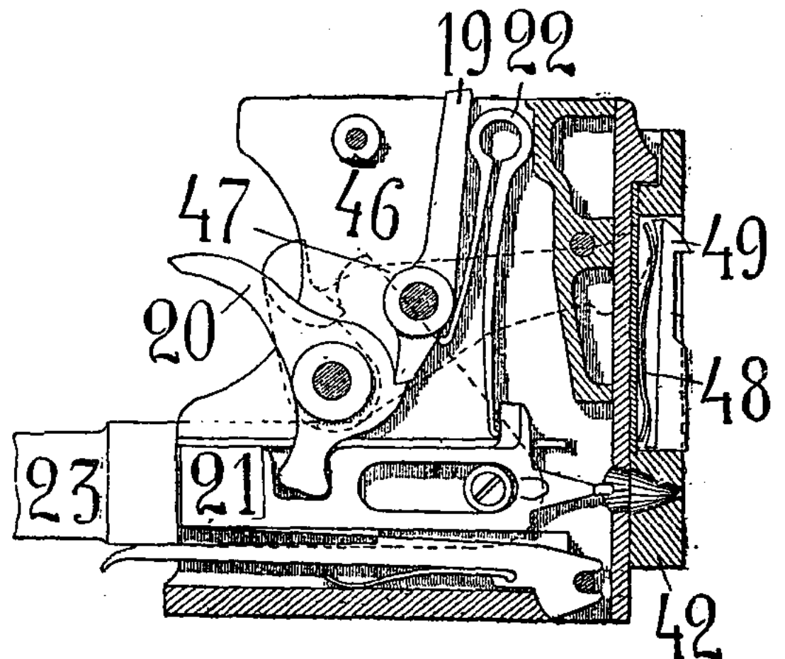
Рис. 4. Замок.
