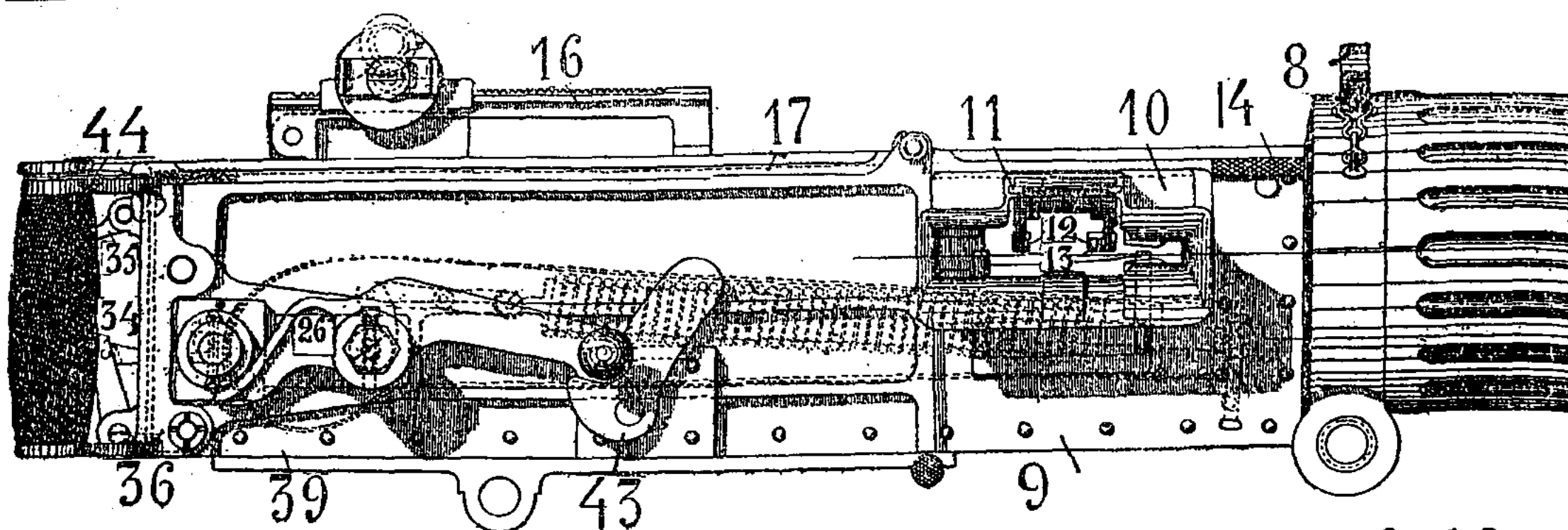
Рис. 1. Вид сбоку.
