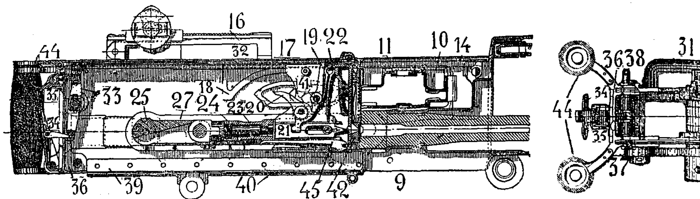
Рис. 2. Продольный разрез.
