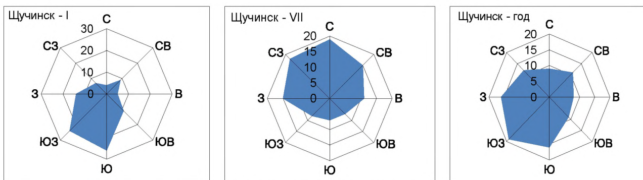
Рисунок 3.15 – Роза ветров на МС Щучинск
