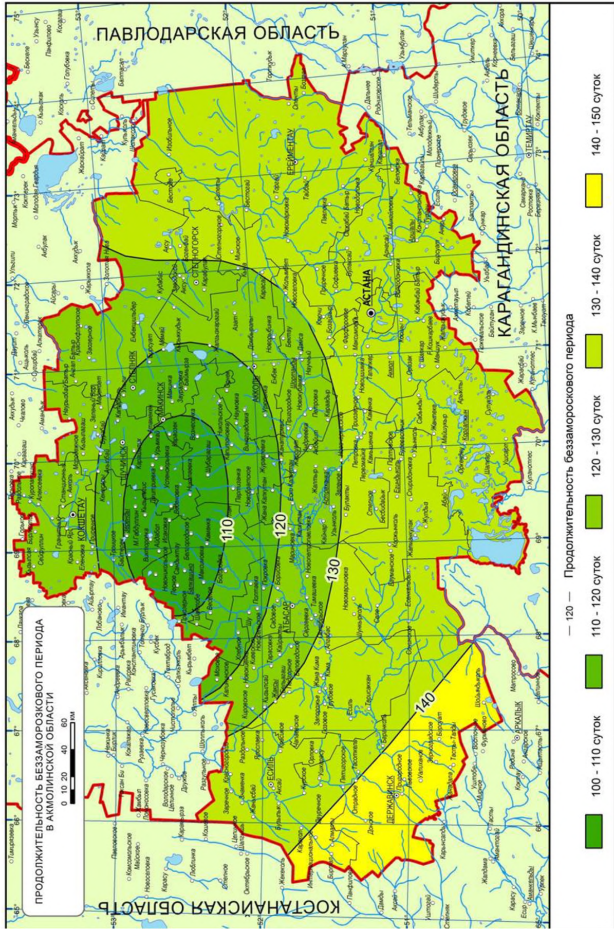
Рисунок 4.4 – Продолжительность беззаморозкового периода в воздухе
