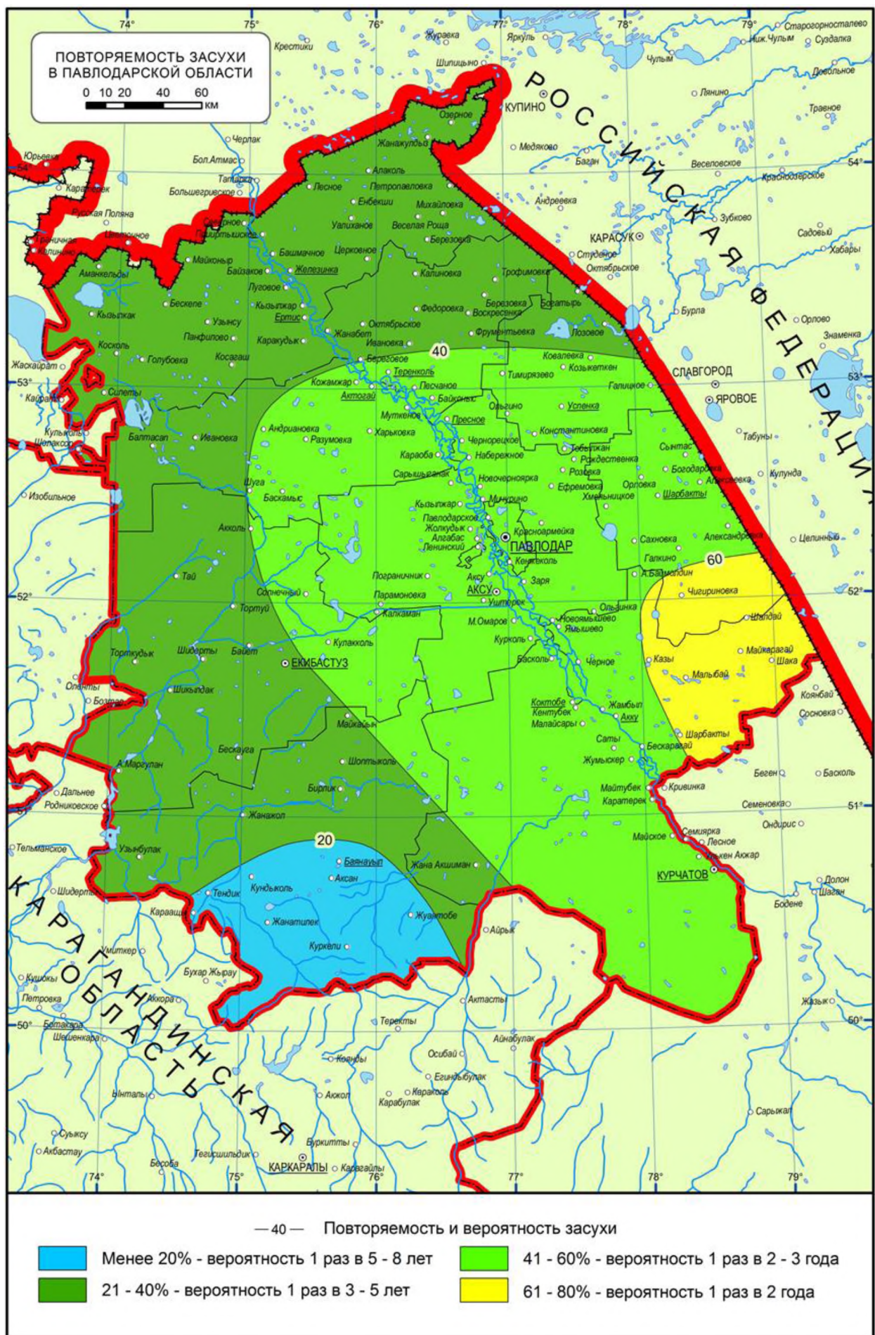
Рисунок 4.1 – Повторяемость засухи
