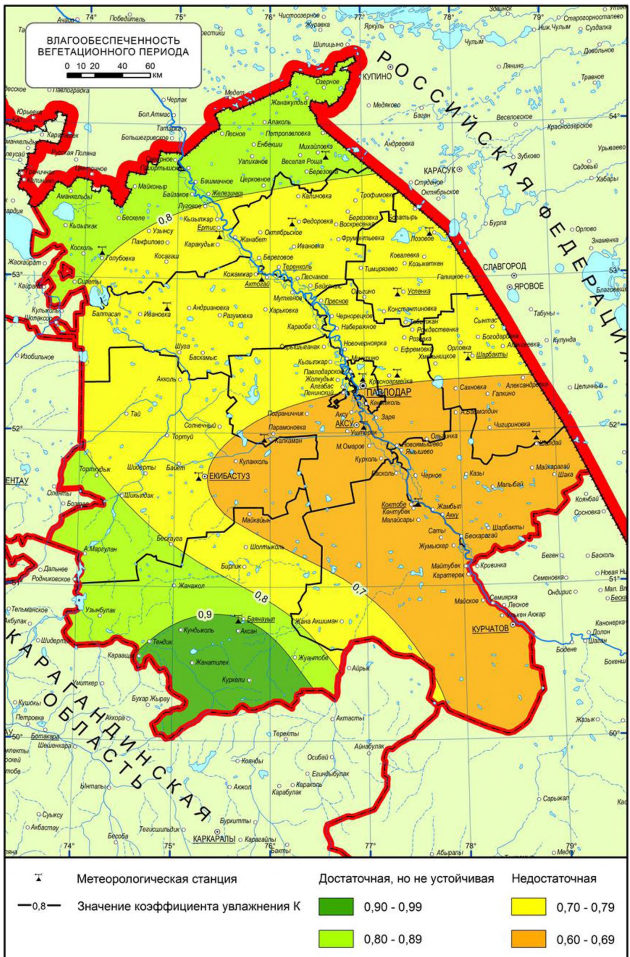
Рисунок 3.10 – Влагообеспеченность вегетационного периода
