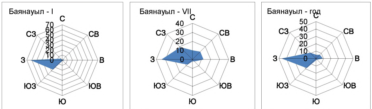
Рисунок 3.18 – Роза ветров на МС Баянауыл
