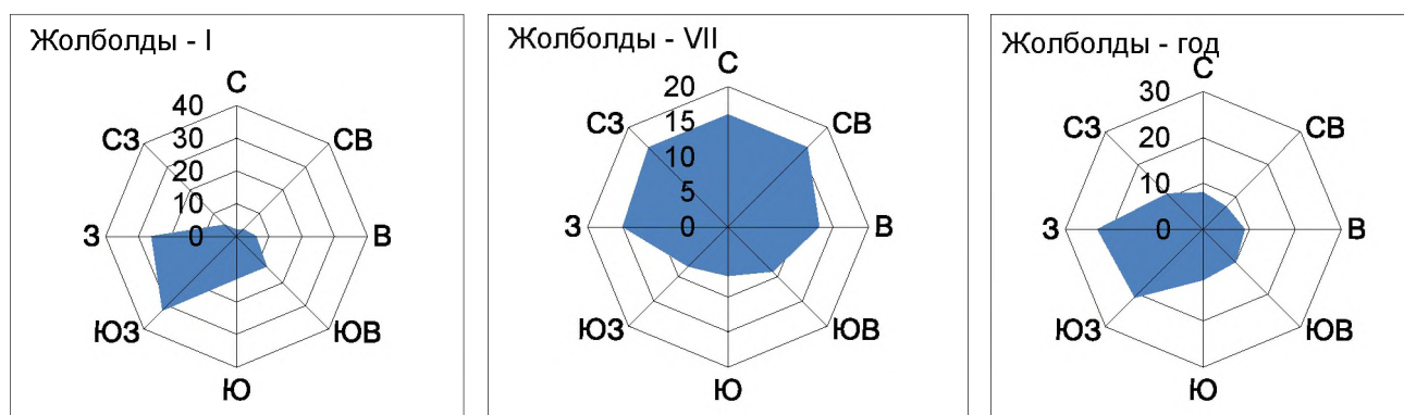
Рисунок 3.16 – Роза ветров на МС Жолболды
