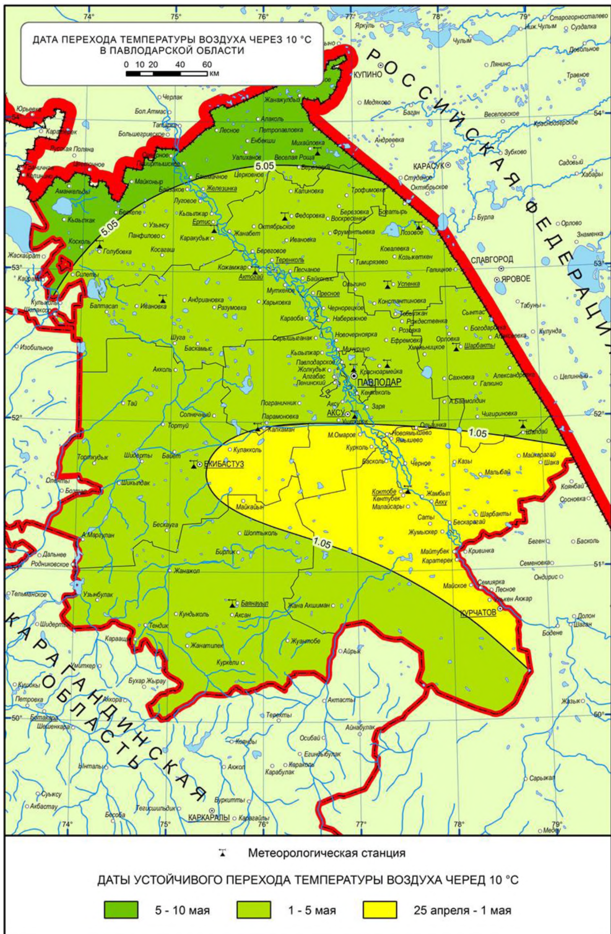
Рисунок 3.4 – Дата устойчивого перехода температуры воздуха через 10°C весной
