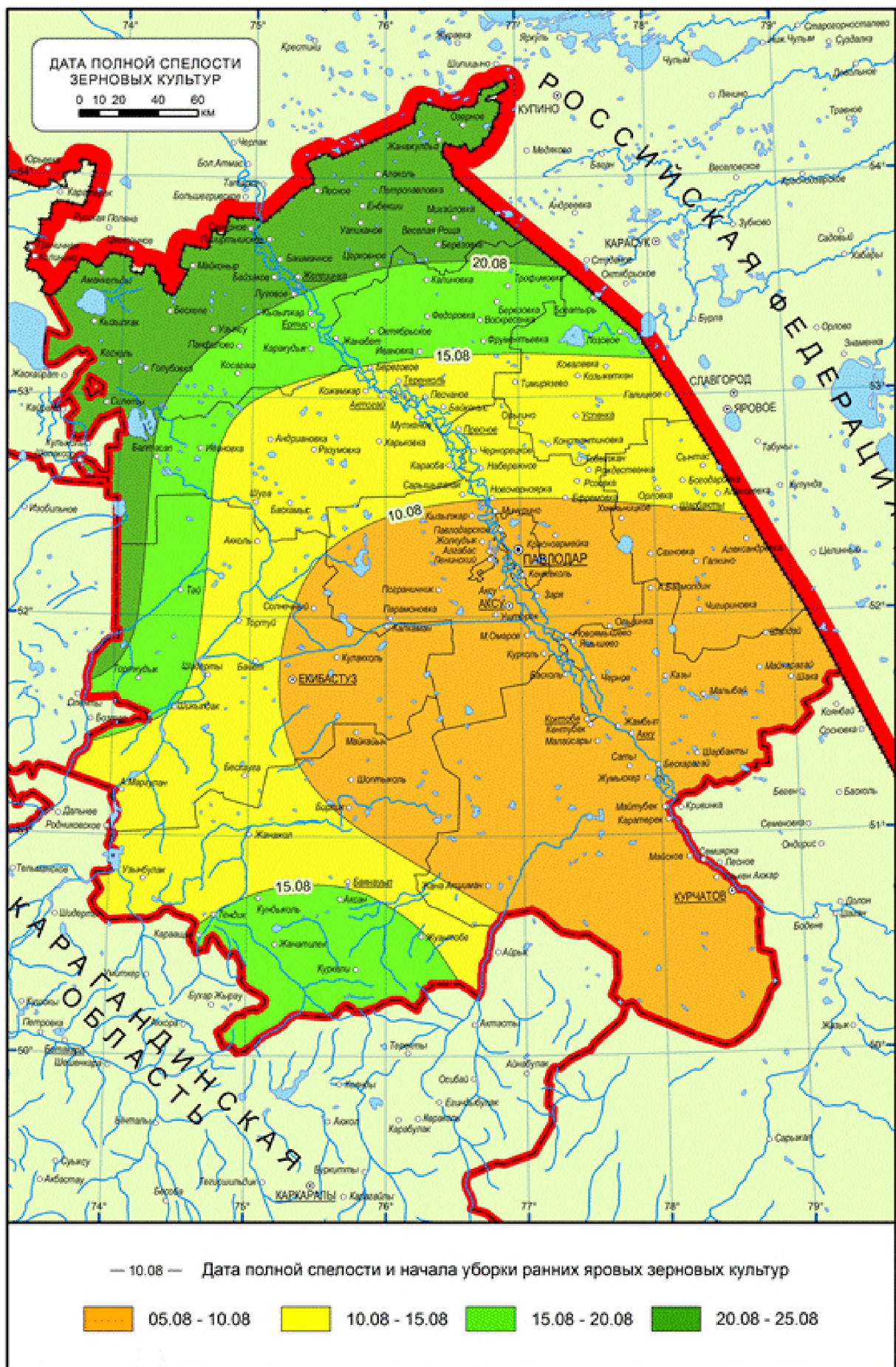
Рисунок 5.3 – Климатические сроки полной спелости и начала уборки ранних яровых зерновых культур
