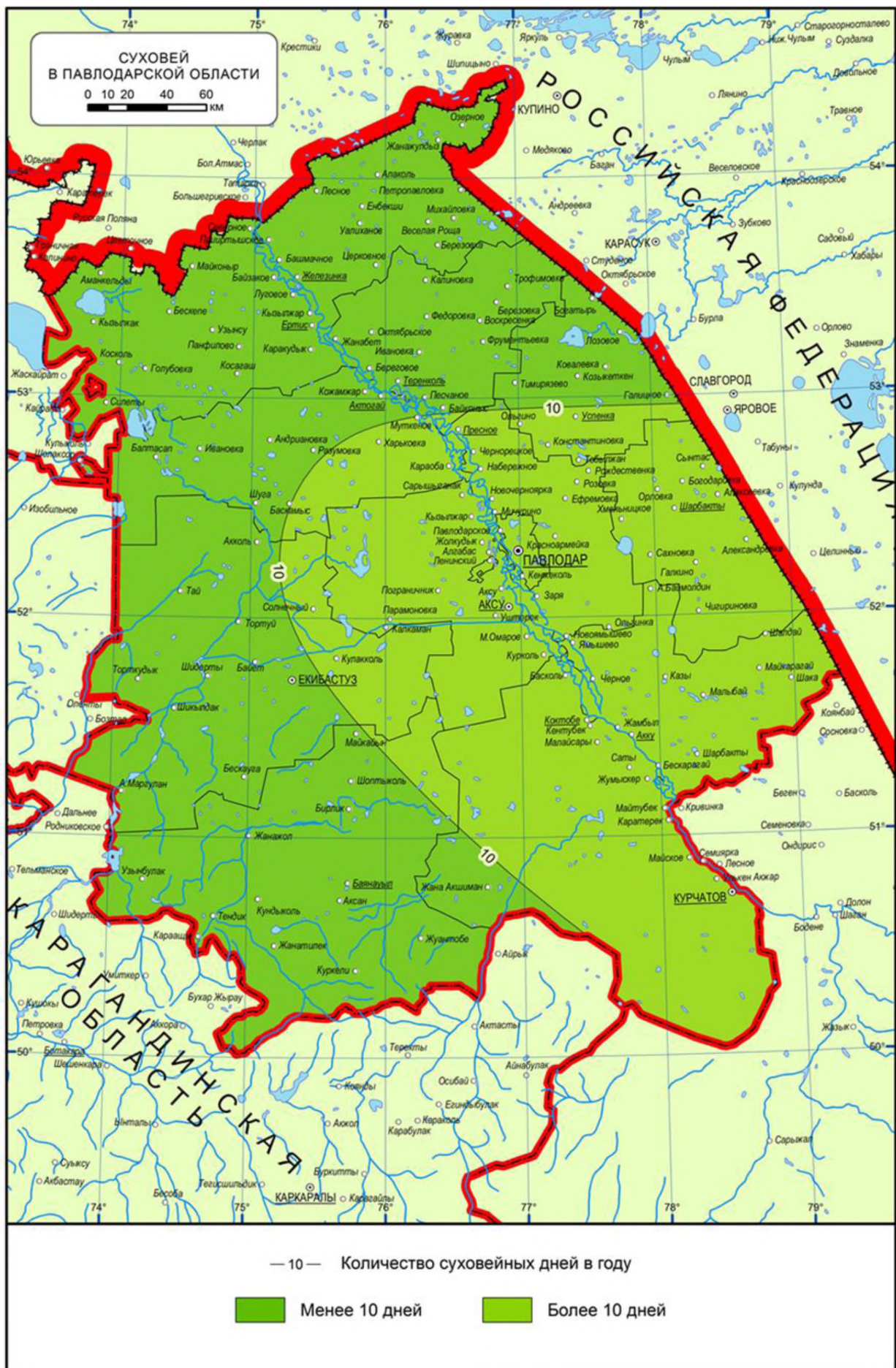
Рисунок 4.3 - Количество дней в году с суховеями умеренной и сильной интенсивности
