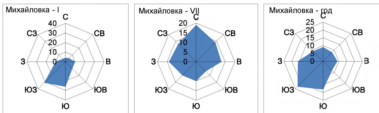
Рисунок 3.15 – Роза ветров на МС Михайловка
