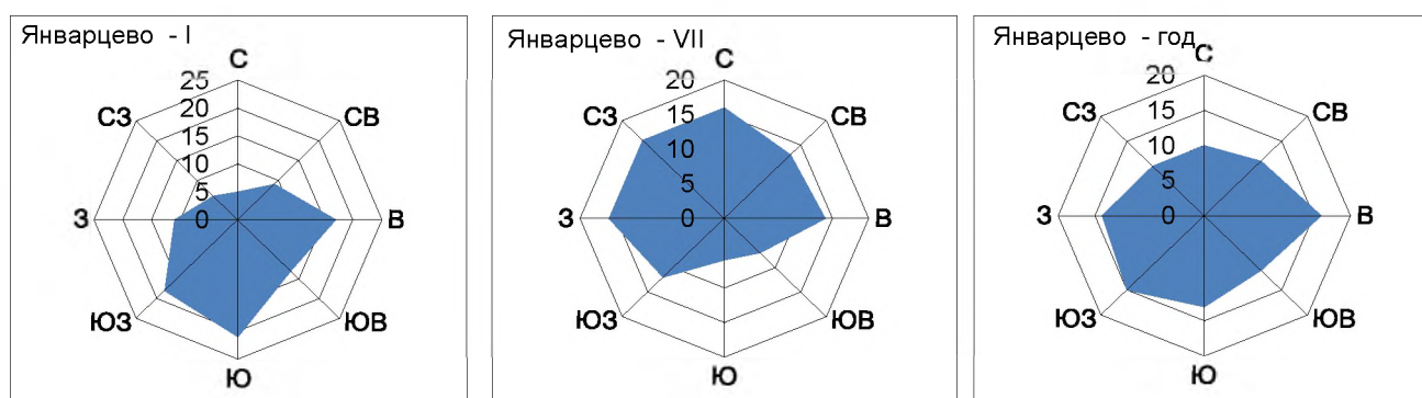
Рисунок 3.15 – Роза ветров на МС Январцево
