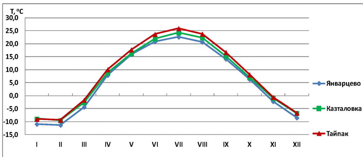
Рисунок 3.3 – Годовой ход средних месячных температур воздуха
