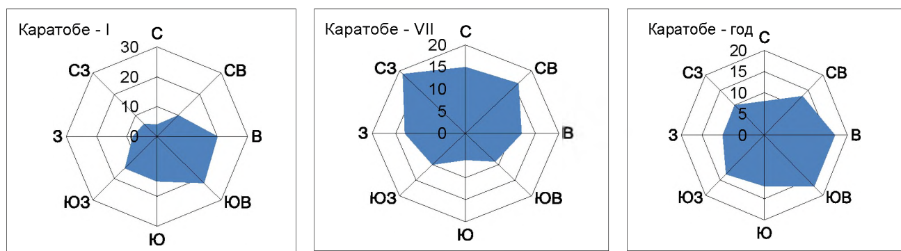
Рисунок 3.17 – Роза ветров на МС Каратобе
