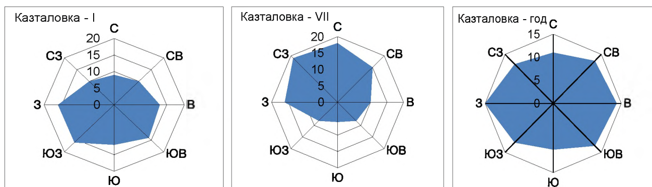
Рисунок 3.16 – Роза ветров на МС Казталовка
