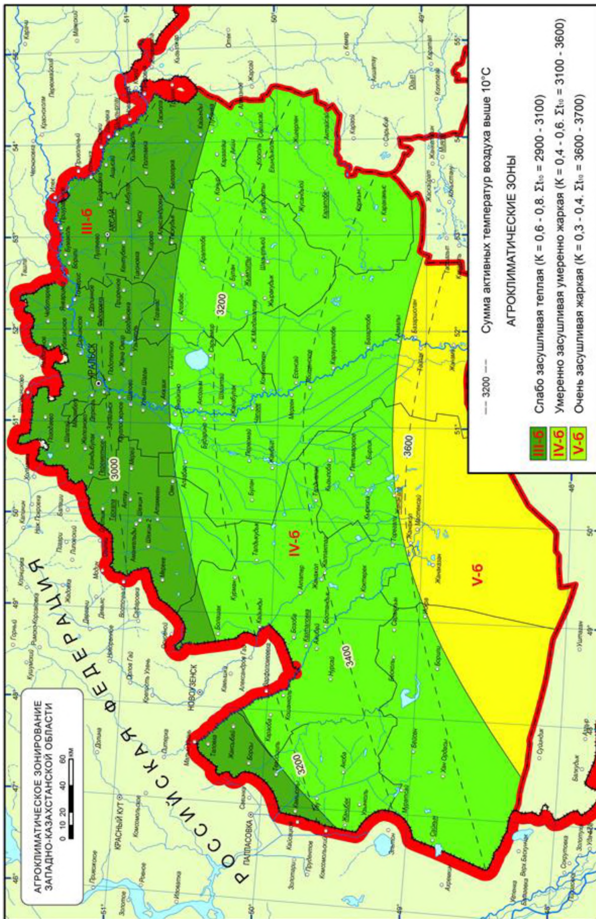
Рисунок 3.2 – Агроклиматическое зонирование территории Западно-Казакстанской области
