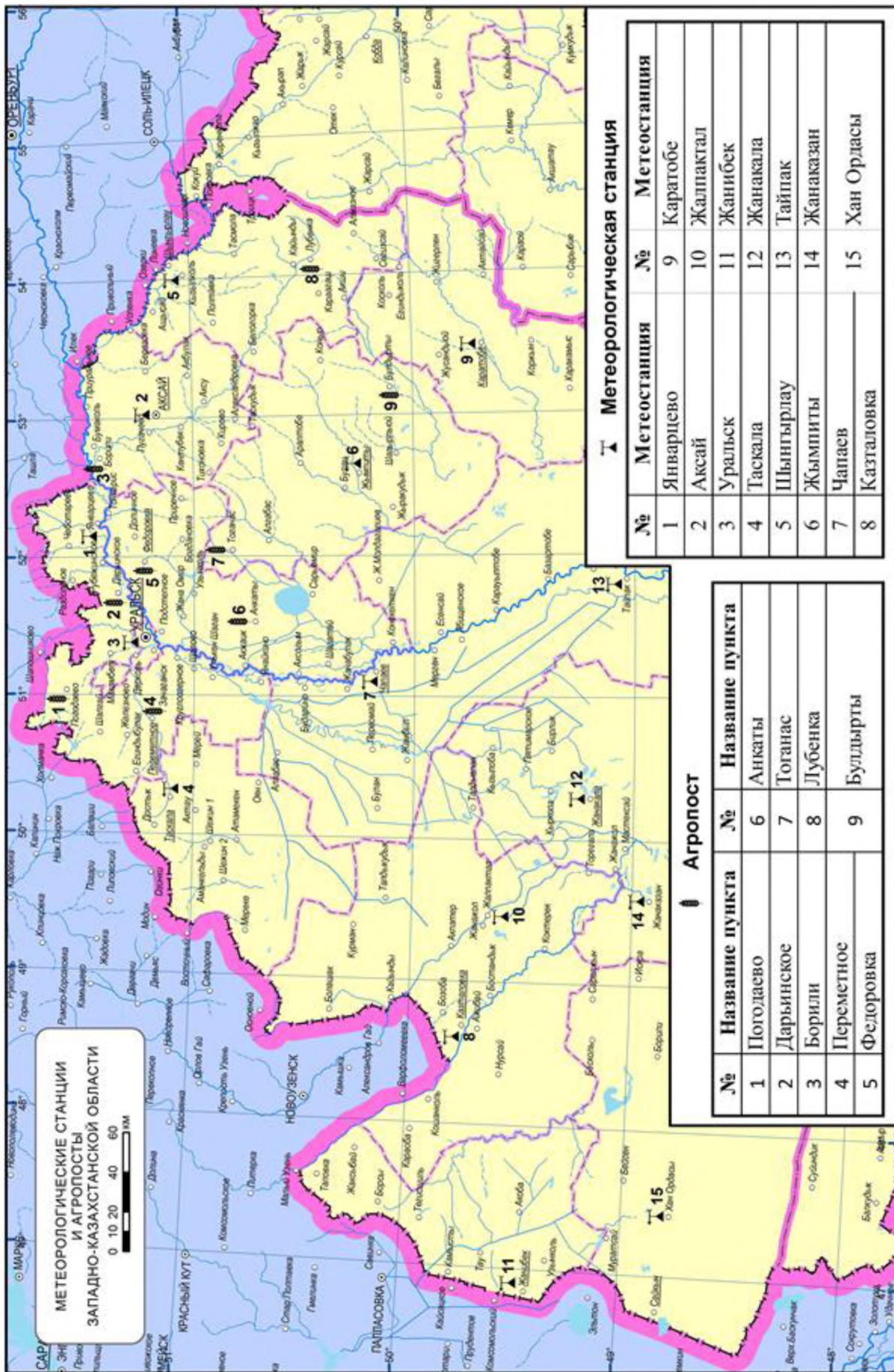
Рисунок 3.1 – Метеорологические станции Западно-Казахстанской области
