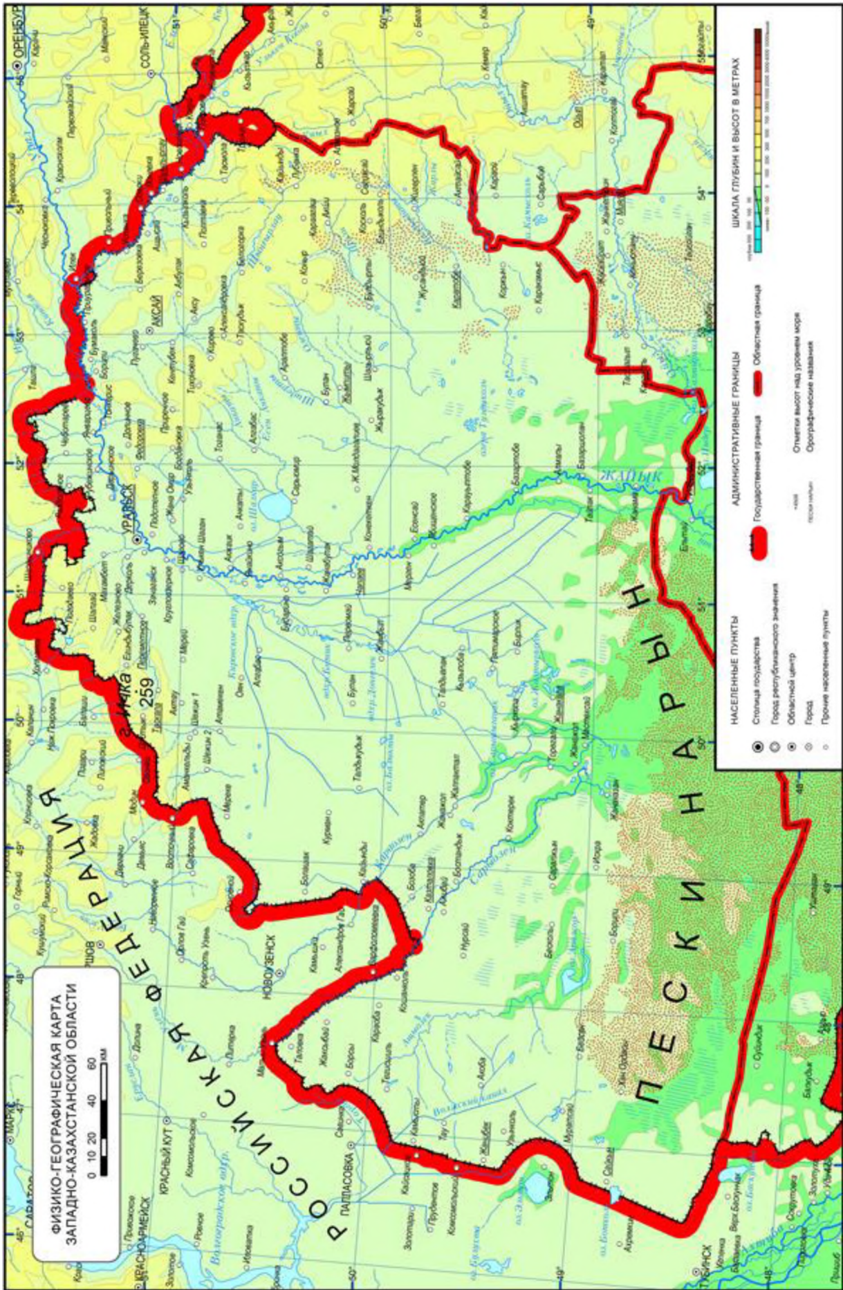
Рисунок 2.2 – Физико-географическая карта Западно-Казакстанской области
