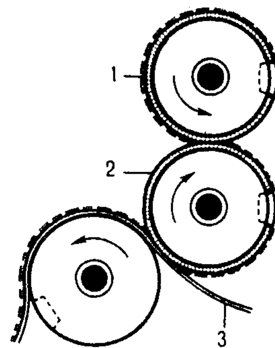
Офсетная печать (схема): 1 — печатная форма; 2 — резиновое полотно; 3 — бумага
